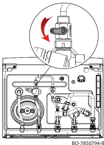
Obr.21 Plnění topného systému
