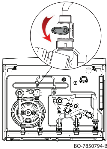
Fig.44 Llenado de la instalación
